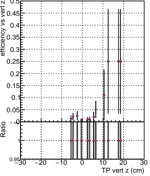
Efficiency vs vert z — DQM mkFit Ximinus NOBU NEWdefault specPLess1 — DQM mkFit Ximinus NOBU NEWdefault specPLess2 — DQM mkFit Ximinus NOBU NEWdefault specPLess3 — DQM mkFit Ximinus NOBU NEWdefault specPLess4
