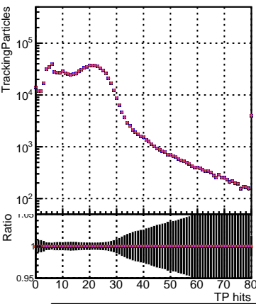
— DQM_mkFit_XiminusNOPU_NEWdefault — DQM_mkFit_XiminusNOPU_NEWdefault_specLess1 — DQM_mkFit_XiminusNOPU_NEWdefault_specLess2 — DQM_mkFit_XiminusNOPU_NEWdefault_specLess3 — DQM_mkFit_XiminusNOPU_NEWdefault_specLess4
