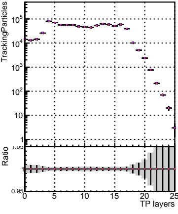
N of sim DQM_mkFit_XiminusNOPU_NEWdefault DQM_mkFit_XiminusNOPU_NEWdefault_specLess1 DQM_mkFit_XiminusNOPU_NEWdefault_specLess2 DQM_mkFit_XiminusNOPU_NEWdefault_specLess3 DQM_mkFit_XiminusNOPU_NEWdefault_specLess4
