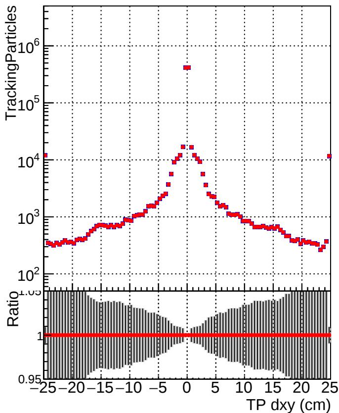
■ DQM_mkFit_XiminusNOPU_NEWdefault ■ DQM_mkFit_XiminusNOPU_OLD6iters
