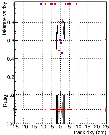
—●— DQM_mkFit_XiminusNOPU_NEWdefault —●— DQM_mkFit_XiminusNOPU_OLD6iters
