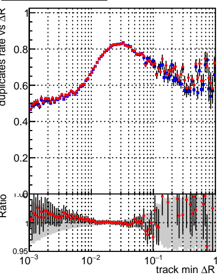
—●— DQM_mkFit_XiminusNOPU_NEWdefault —●— DQM_mkFit_XiminusNOPU_OLD6iters
