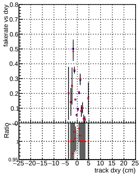
—●— DQM_mkFit_XiminusNOPU_NEWdefault —●— DQM_mkFit_XiminusNOPU_OLD6iters
