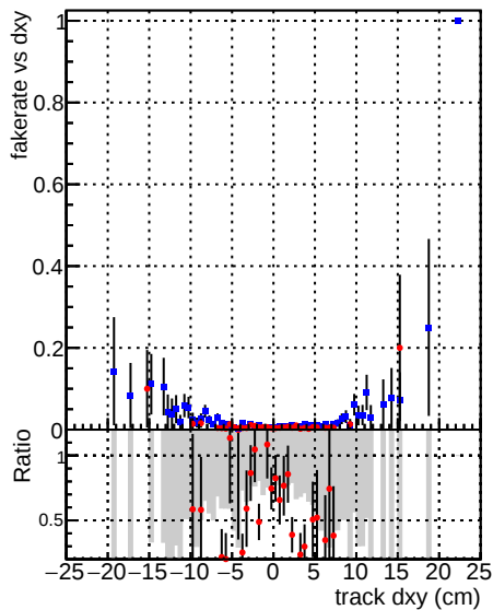
—●— DQM_mkFit_XiminusNOPU_NEWdefault —●— DQM_mkFit_XiminusNOPU_OLD6iters
