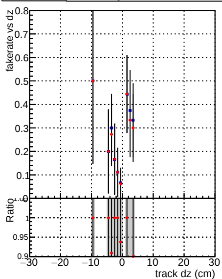
— DQM_mkFit_XiminusNOPU_NEWdefault — DQM_mkFit_XiminusNOPU_OLD6iters
