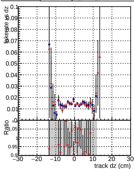
— DQM_mkFit_XiminusNOPU_NEWdefault — DQM_mkFit_XiminusNOPU_OLD6iters
