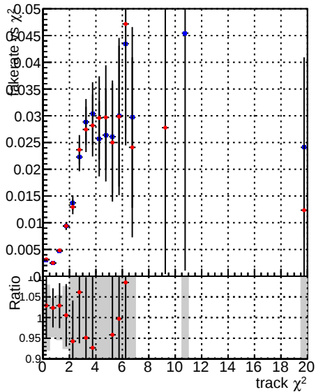
Fake rate vs. —•— DQM_mkFit_XiminusNOPU_NEWdefault —•— DQM_mkFit_XiminusNOPU_OLD6iters
