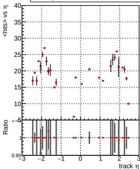
— DQM_mkFit_XiminusNOPU_NEWdefault — DQM_mkFit_XiminusNOPU_OLD6iters
