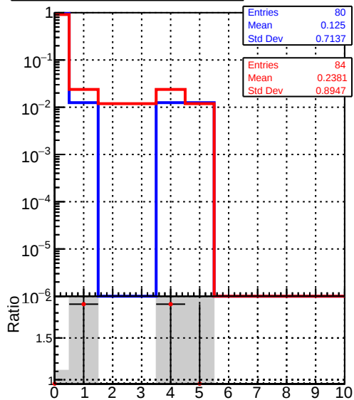
— DQM_mkFit_XiminusNOPU_NEWdefault — DQM_mkFit_XiminusNOPU_OLD6iters
