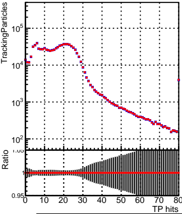
■ DQM_mkFit_XiminusNOPU_NEWdefault ■ DQM_mkFit_XiminusNOPU_OLD6iters
