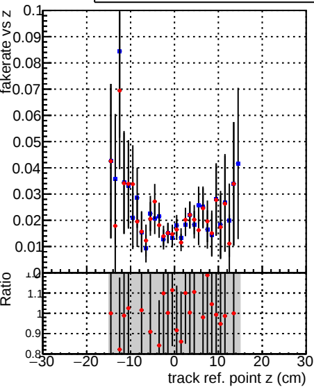
Fake rate vs verpos —●— DQM_mkFit_XiminusNOPU_NEWdefault —●— DQM_mkFit_XiminusNOPU_OLD6iters
