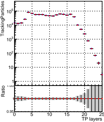
DQM_mkFit_XiminusNOPU_NEWdefault
