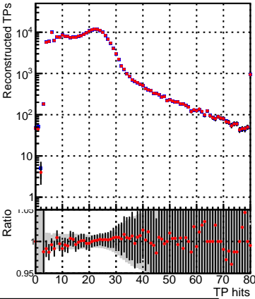
DQM_mkFit_XiminusNOPU_OLD6iters
