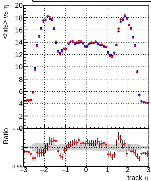
mean hits — DQM_mkFit_XiminusNOPU_NEWdefault — DQM_mkFit_XiminusNOPU_OLD6iters
