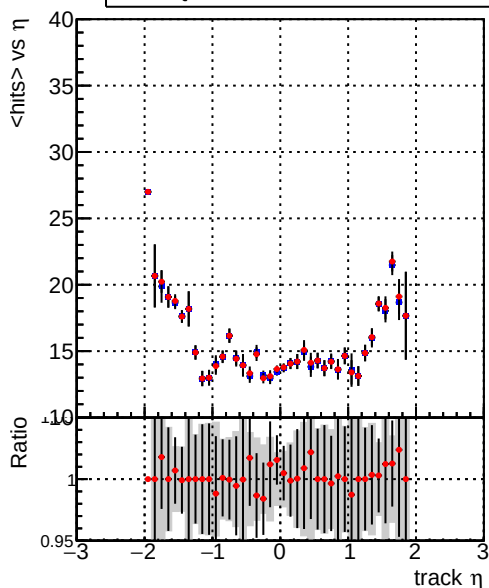
mean hits — DQM_mkFit_XiminusNOPU_NEWdefault — DQM_mkFit_XiminusNOPU_OLD6iters
