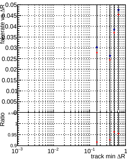
Fake rate vs \Delta R(\text{track, jet}) DQM_mkFit_XiminusNOPU_NEWdefault DQM_mkFit_XiminusNOPU_OLD6iters
