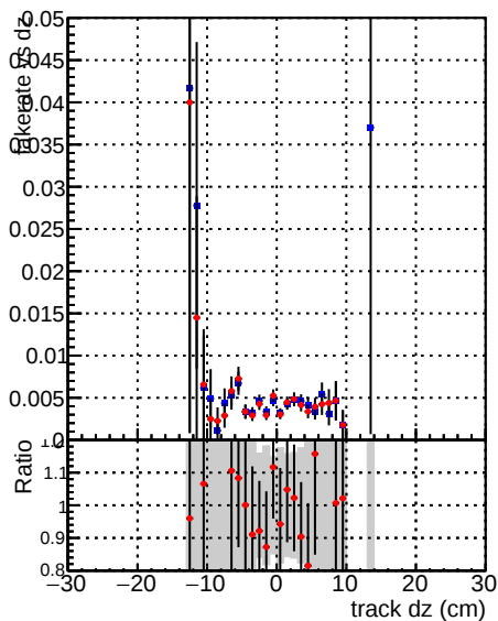
—●— DQM_mkFit_XiminusNOPU_NEWdefault —●— DQM_mkFit_XiminusNOPU_OLD6iters
