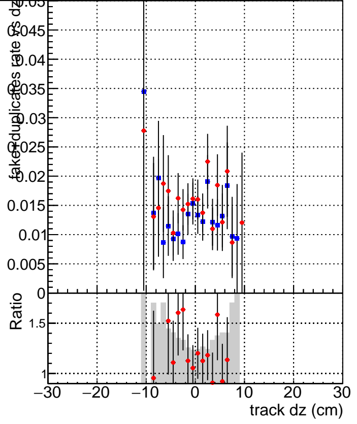
DQM_mkFit_XiminusNOPU_NEWdefault DQM_mkFit_XiminusNOPU_OLD6iters
