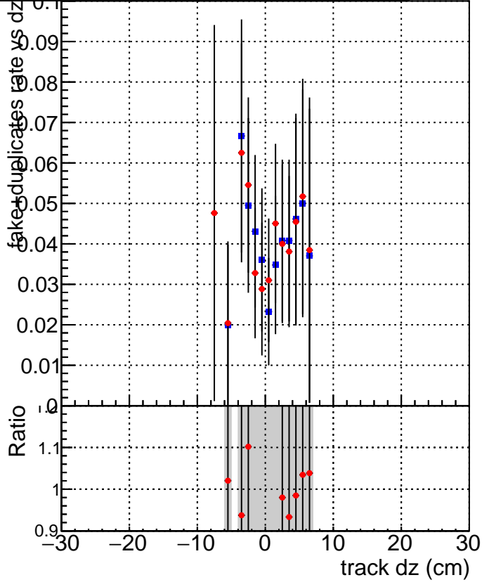
DQM_mkFit_XiminusNOPU_NEWdefault DQM_mkFit_XiminusNOPU_OLD6iters
