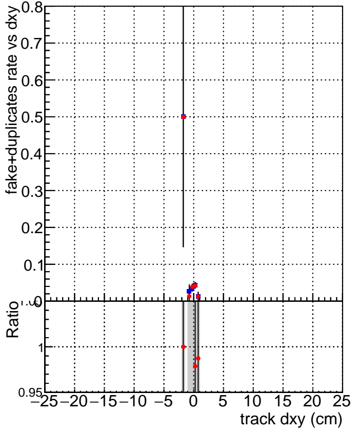
DQM_mkFit_XiminusNOPU_NEWdefault DQM_mkFit_XiminusNOPU_OLD6iters
