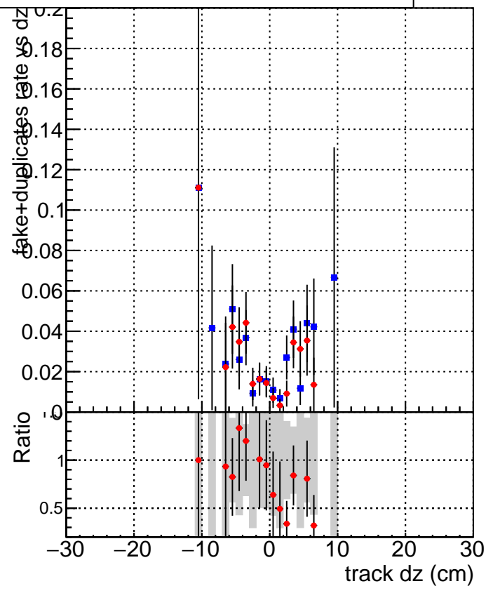
DQM_mkFit_XiminusNOPU_NEWdefault DQM_mkFit_XiminusNOPU_OLD6iters
