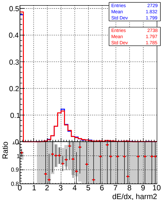
■ DQM_mkFit_XiminusNOPU_NEWdefault ● DQM_mkFit_XiminusNOPU_OLD6iters
