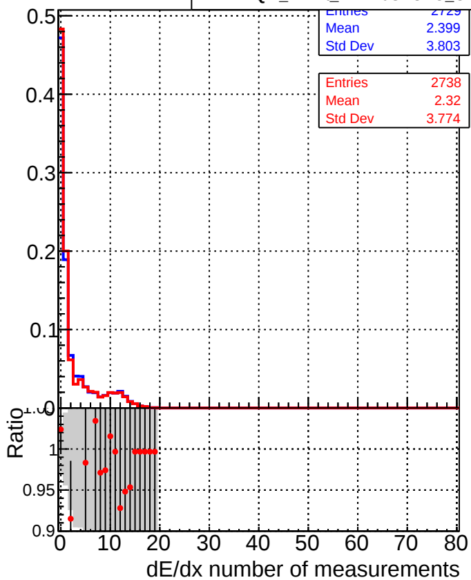
■ DQM_mkFit_XiminusNOPU_NEWdefault ● DQM_mkFit_XiminusNOPU_OLD6iters
