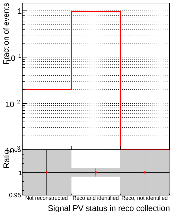
DQM_mkFit_XiminusNOPU_NEWdefault DQM_mkFit_XiminusNOPU_OLD6iters
