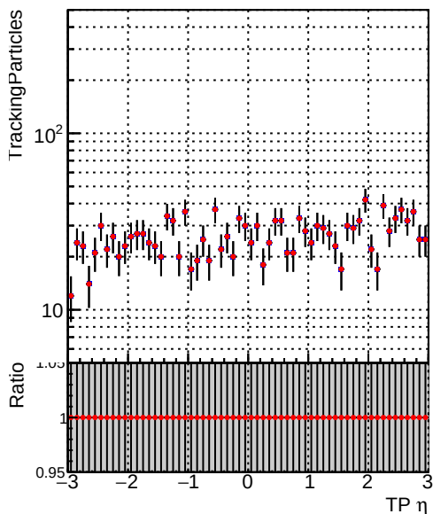
N of sin —●— DQM_mkFit_XiminusNOPU_OLD6iters
