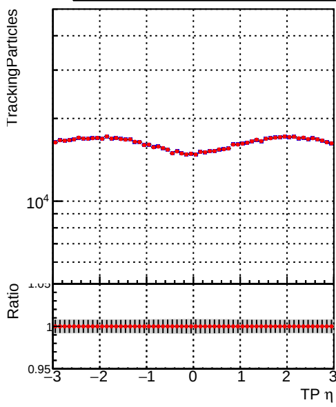
—•— DQM_mkFit_XiminusNOPU_NEWdefault —•— DQM_mkFit_XiminusNOPU_OLD6iters
