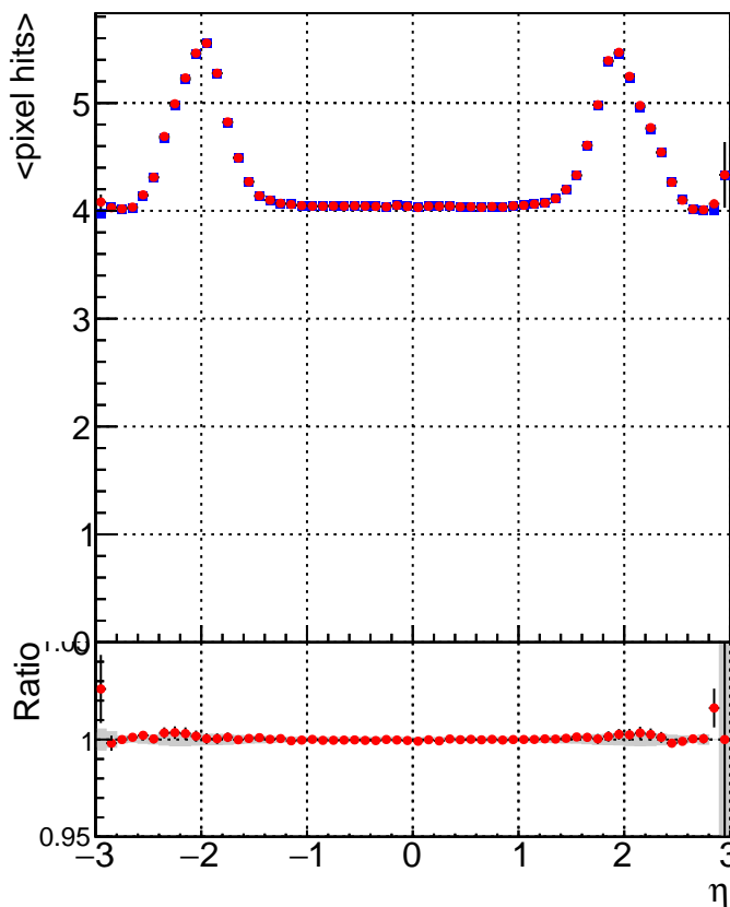
■ DQM_mkFit_XiminusNOPU_NEWdefault ■ DQM_mkFit_XiminusNOPU_OLD6iters
