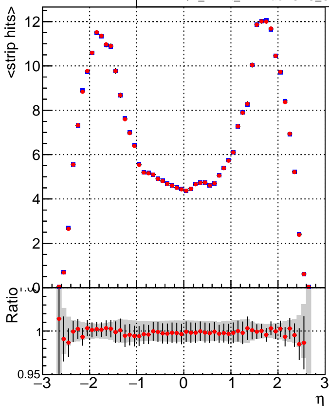
■ DQM_mkFit_XiminusNOPU_NEWdefault ■ DQM_mkFit_XiminusNOPU_OLD6iters
