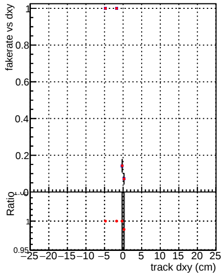
— DQM_mkFit_XiminusNOPU_NEWdefault — DQM_mkFit_XiminusNOPU_OLD6iters
