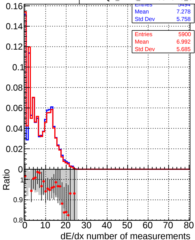
—■— DQM_mkFit_XiminusNOPU_NEWdefault —●— DQM_mkFit_XiminusNOPU_OLD6iters
