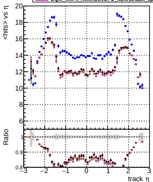
Legend: DQM mkFit XiMinusNOPU NEWdefault specPless1 (blue), DQM mkFit XiMinusNOPU NEWdefault specPless2 (red), DQM mkFit XiMinusNOPU NEWdefault specPless3 (orange), DQM mkFit XiMinusNOPU NEWdefault specPless4 (purple) mean hits vs \eta
