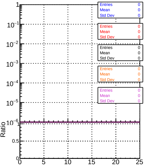
mean hit Legend: DQM mkFit XiMinusNOPU NEWdefault specPless1 (blue), DQM mkFit XiMinusNOPU NEWdefault specPless3 (red), DQM mkFit XiMinusNOPU NEWdefault specPless4 (orange), DQM mkFit XiMinusNOPU NEWdefault specPless2 (purple)
