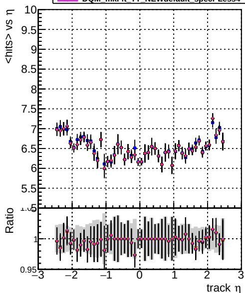
Legend: DQM mkFit TT NEWdefault specPLess1 (blue), DQM mkFit TT NEWdefault specPLess2 (red), DQM mkFit TT NEWdefault specPLess3 (orange), DQM mkFit TT NEWdefault specPLess4 (purple) mean hits
