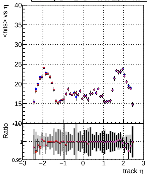
mean hit DQM mkFit TT (tau) NEWdefault specPless1 DQM mkFit TT NEWdefault specPless2 DQM mkFit TT NEWdefault specPless3 DQM mkFit TT NEWdefault specPless4
