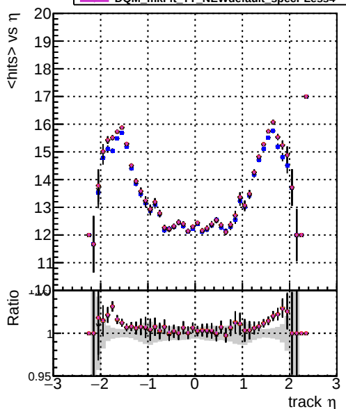
mean hit DQM mkFit TT (tau) NEWdefault specPLess1 DQM mkFit TT (tau) NEWdefault specPLess2 DQM mkFit TT (tau) NEWdefault specPLess3 DQM mkFit TT (tau) NEWdefault specPLess4
