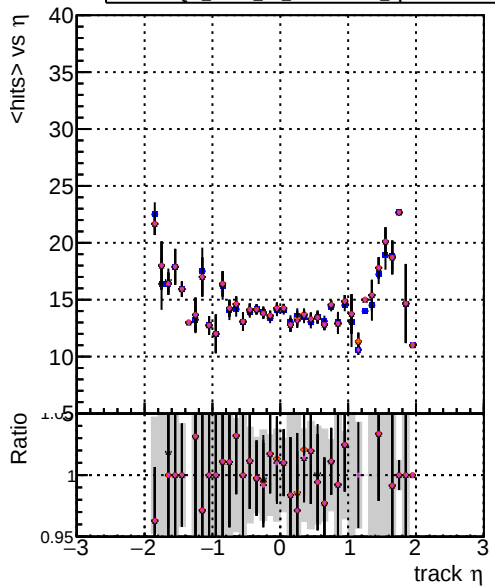
mean hit DQM mkFit TT (draw) NEWdefault specPless1 DQM mkFit TT NEWdefault specPless2 DQM mkFit TT NEWdefault specPless3 DQM mkFit TT NEWdefault specPless4
