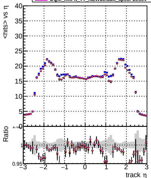
Legend: DQM mkFit TT NEWdefault specPless1, DQM mkFit TT NEWdefault specPless2, DQM mkFit TT NEWdefault specPless3, DQM mkFit TT NEWdefault specPless4 mean hits
