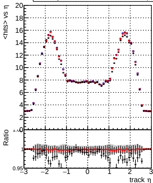
mean hits — DQM_mkFit_baseline_lowPT — DQM_mkFit_baseline6iter_lowPT — DQM_mkFit_TT_RetrainV2_WP2_6iter_ep3_lowPT
