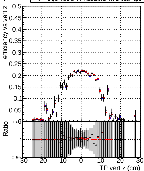
Efficiency vs vert z — DQM_mkFit_baseline_lowPT — DQM_mkFit_baseline6iter_lowPT — DQM_mkFit_TT_RetrainV2_WP2_6iter_ep3_lowPT
