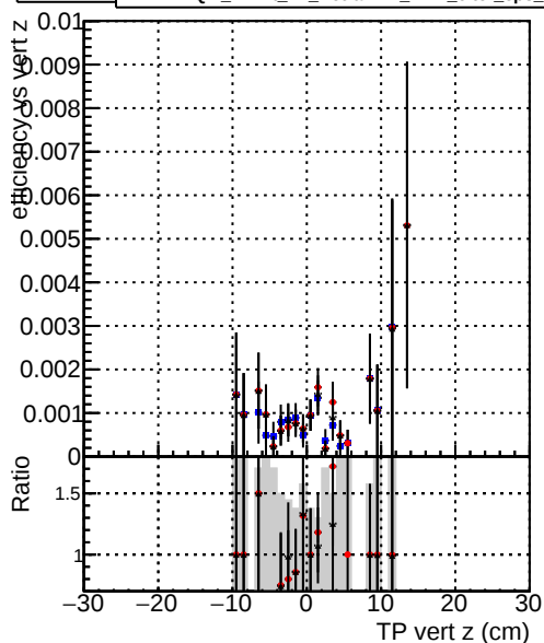
Efficiend —●— DQM_mkFit_baseline6iter_lowPT —▲— DQM_mkFit_TT_RetrainV2_WP2_6iter_ep3_lowPT
