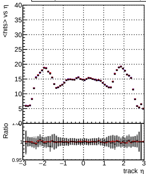
mean hits — DQM_mkFit_baseline_lowPT — DQM_mkFit_baseline6iter_lowPT — DQM_mkFit_TT_RetrainV2_WP2_6iter_ep3_lowPT
