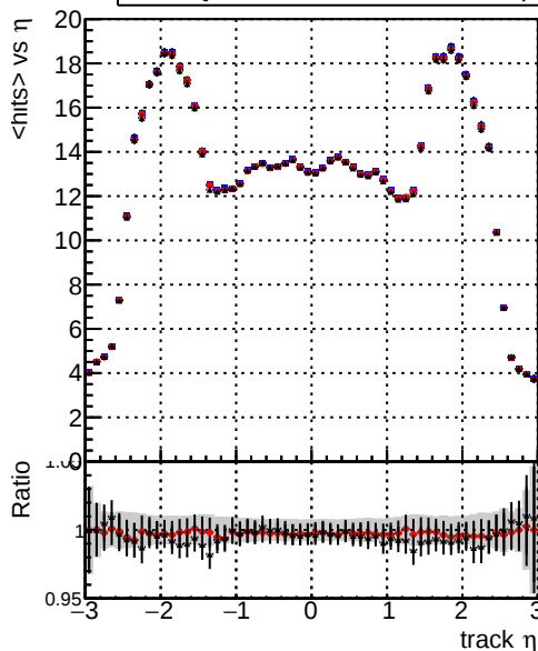
mean hit — DQM_mkFit_baseline_lowPT — DQM_mkFit_baseline6iter_lowPT — DQM_mkFit_TT_RetrainV2_WP2_6iter_ep3_lowPT
