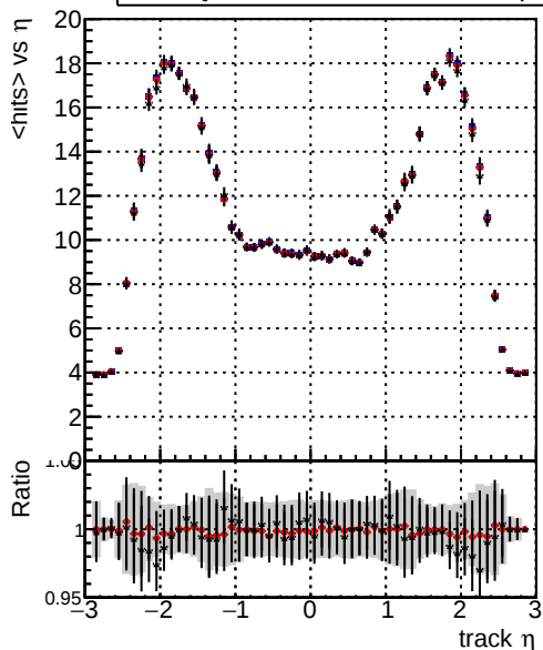
mean hit — DQM_mkFit_baseline_lowPT — DQM_mkFit_baseline6iter_lowPT — DQM_mkFit_TT_RetrainV2_WP2_6iter_ep3_lowPT
