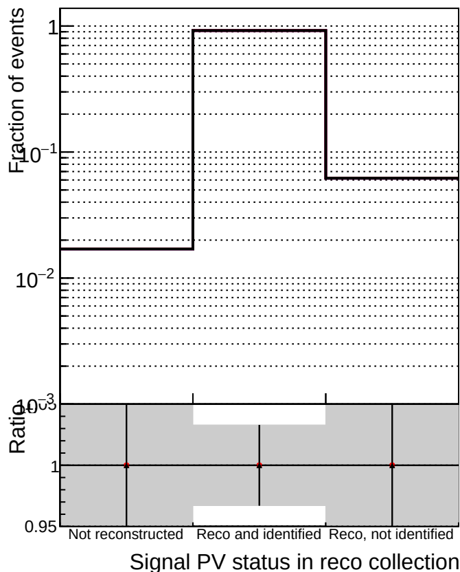
—■ DQM_mkFit_baseline_lowPT —● DQM_mkFit_baseline6iter_lowPT —■ DQM_mkFit_TT_RetrainV2_WP2_6iter_ep3_lowPT
