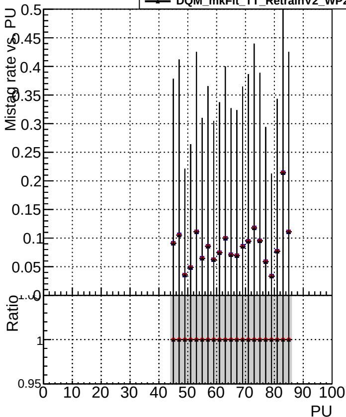
—■ DQM_mkFit_baseline_lowPT —● DQM_mkFit_baseline6iter_lowPT —■ DQM_mkFit_TT_RetrainV2_WP2_6iter_ep3_lowPT
