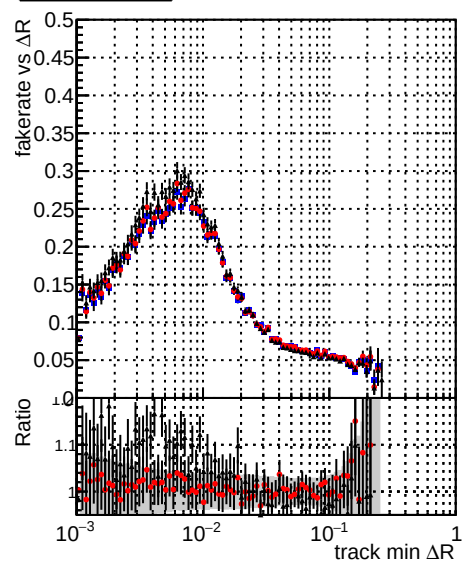
—●— DQM mkFit baseline_lowPT —●— DQM mkFit baseline6iter_lowPT —●— DQM mkFit TT_RetrainV2_LP2_6iter_ep3_lowPT
