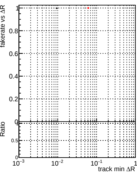
Legend: —●— DQM_mkFit_baseline_lowPT —●— DQM_mkFit_baseline6iter_lowPT —●— DQM_mkFit_TT_RetrainV2_WP2_6iter_ep3_lowPT
