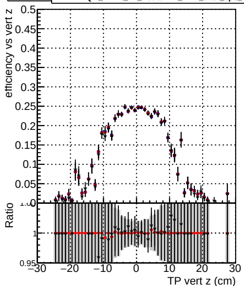
Efficiency vs. TP vert z (cm) — DQM_mkFit_baseline_lowPT — DQM_mkFit_baseline6iter_lowPT — DQM_mkFit_TT_RetrainV2_WP2_6iter_ep3_lowPT
