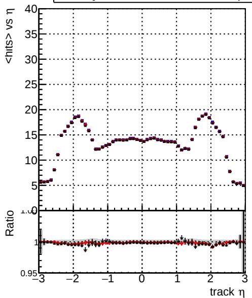
DQM_mkFit_baseline_lowPT DQM_mkFit_baseline6iter_lowPT DQM_mkFit_TT_RetrainV2_WP2_6iter_ep3_lowPT mean hits
