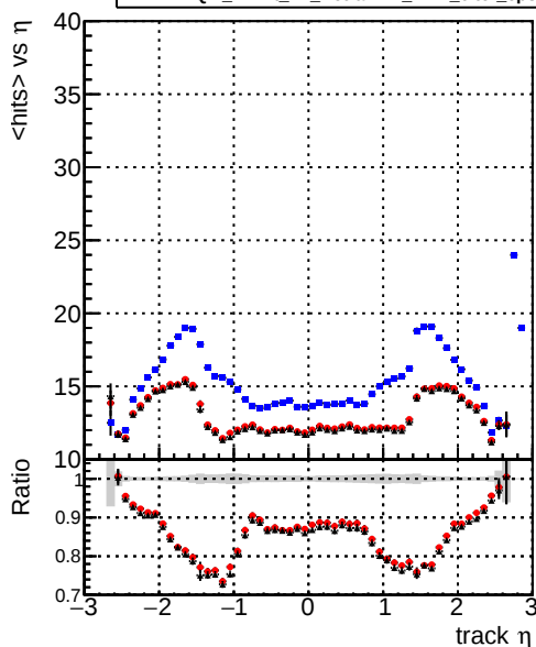
— DQM_mkFit_baseline_lowPT — DQM_mkFit_baseline6iter_lowPT — DQM_mkFit_TT_RetrainV2_WP1_6iter_ep3_lowPT
