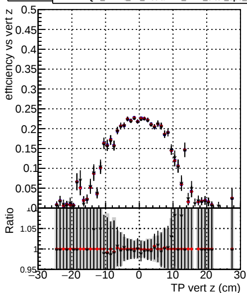
Efficiency vs vert z — DQM_mkFit_baseline_lowPT — DQM_mkFit_baseline6iter_lowPT — DQM_mkFit_TT_RetrainV2_WP1_6iter_ep3_lowPT
