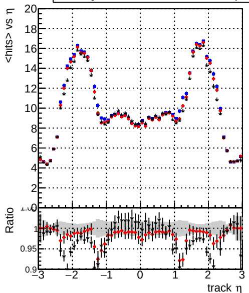
mean hits — DQM_mkFit_baseline_lowPT — DQM_mkFit_baseline6iter_lowPT — DQM_mkFit_TT_RetrainV2_WP1_6iter_ep3_lowPT
